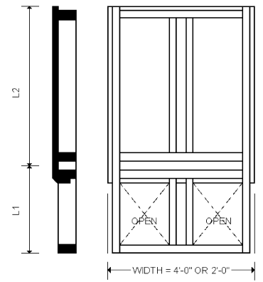
PERGOLA PANEL: #P (W X L1 + L2)
